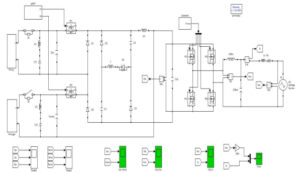
Fig.4.1.Simulation circuit.
