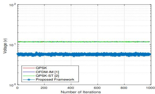
(d) PAPR for 8*8 Antenna Array
