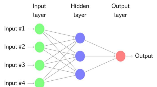
Fig.2 CNN Layer
